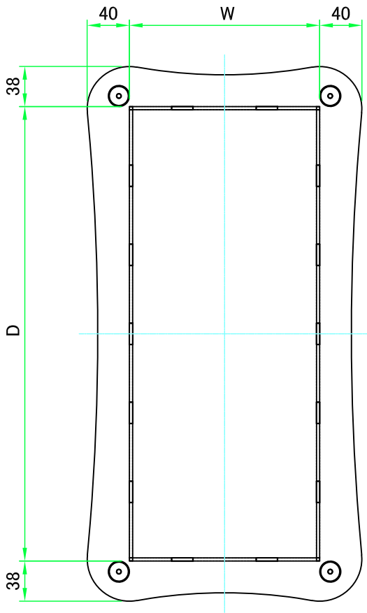
上カバー / Top cover
