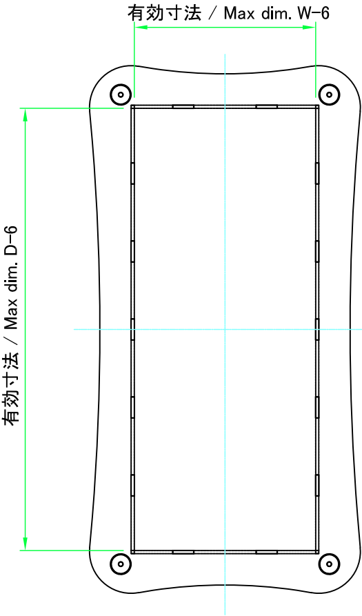
下カバー / Bottom cover
